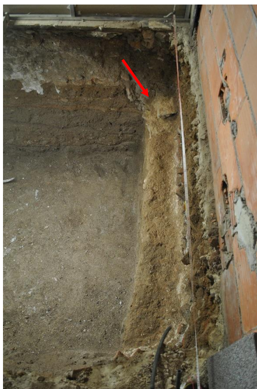
Figs 10 i 11.- La UE 108 en exposició un cop extreta la preparació UE 107. La fletxa assenyalava la UE 110 de la FS01. A dalt, vista des del Sudoest, a la dreta, vista des del Sud.
